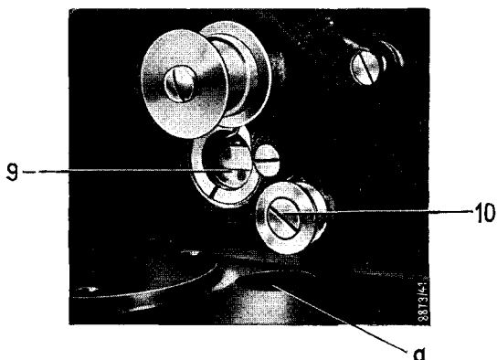
Abb. 12 Oelstandglas und Oelablaß-Stelle
