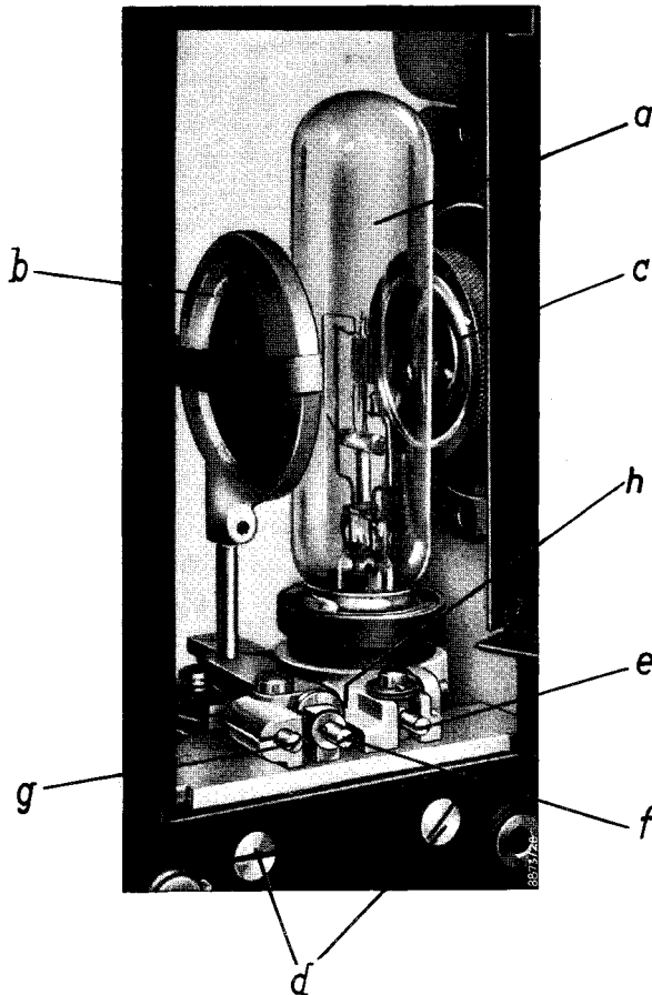
Abb. 7 Lampensystem
