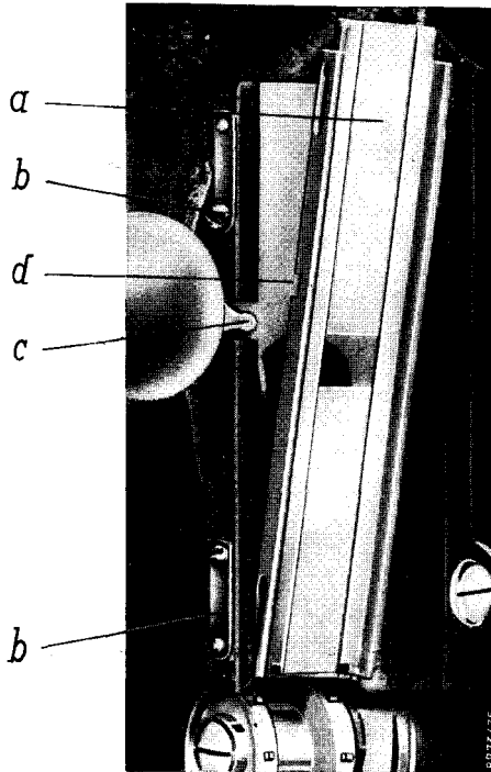
Abb. 14 Filmbahn, Grundplatte abgehoben
