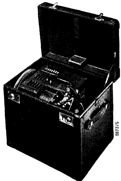
Abb. 16 Selecton im Transportkoffer Gewicht mit Apparat 20 kg Abmessungen 42×30×44 cm
