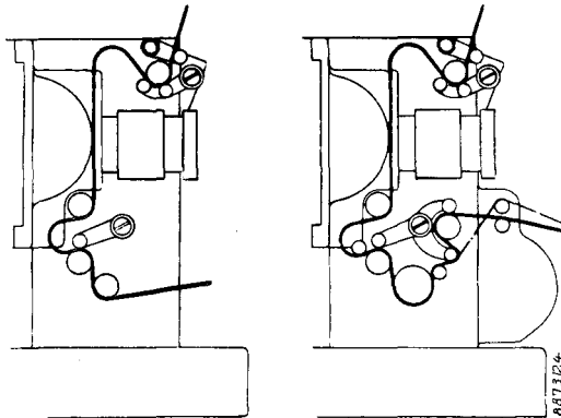
Abb. 3 Filmweg, links für Stummfilm, rechts für Tonfilm
