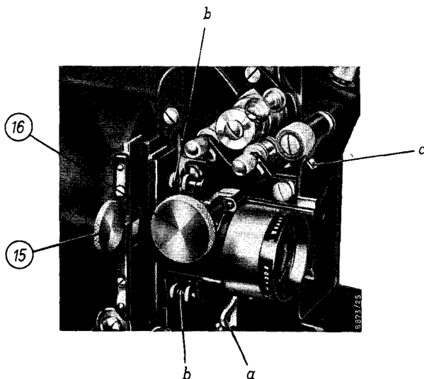
Abb. 4 Filmtüre und Vorwickelrolle
